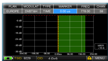
Fig. 1: OTTIMA RICEZIONE: * nessun ECO presente né all'interno né all'esterno della nostra maschera dell'Intervallo di Guardia (area verde).
