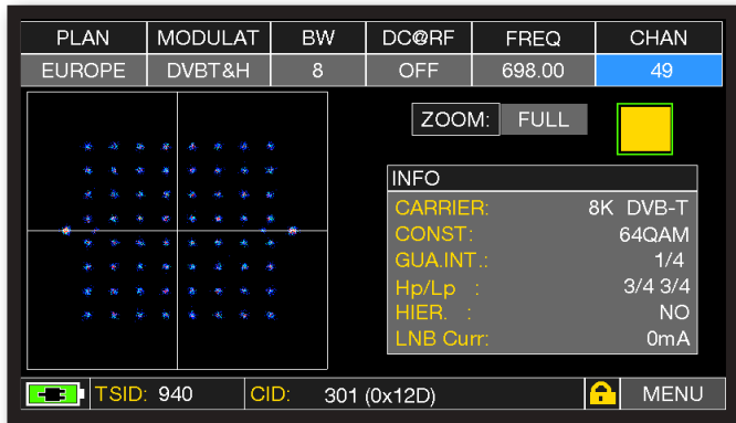
Costellazione DVB-T
