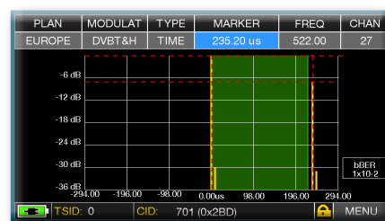
Fig. 3: RICEZIONE MARGINALE (o IMPOSSIBILE):* 2 ECHI presenti all'esterno della maschera dell'Intervallo di Guardia, provenienti da una distanza di: 1° eco: 70,56 Km, pari ad un ritardo di 232,20 \mu s .
