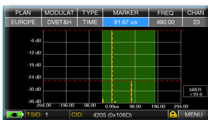
Fig. 2: BUONA RICEZIONE: * 2 ECHI presenti, ma all'interno della maschera nell'Intervallo di Guardia, provenienti da una distanza di: 1° eco: 24,50 Km, pari ad un ritardo di 81,67 \mu s .
