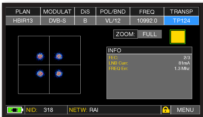
Costellazione QPSK.
