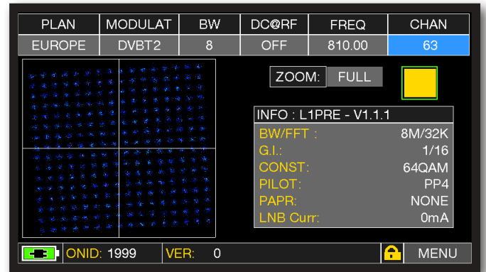
Costellazione DVB-T2
